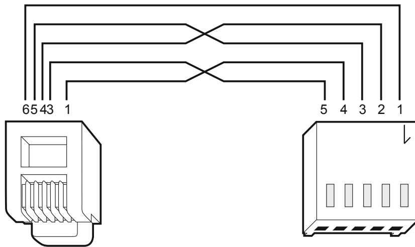
Rys. 13. Sposób połączenia portów RS-232 centrali i modemu zewnętrznego z gniazdem PIN5 (analogicznie podłącza się moduł ETHM-1 / ETHM-1 Plus i moduły GSM firmy SATEL). Po lewej wtyk RJ podłączany do gniazda na płycie głównej centrali. Po prawej wtyk PIN5. Gotowy kabel jest oferowany przez firmę SATEL (RJ/PIN5).
