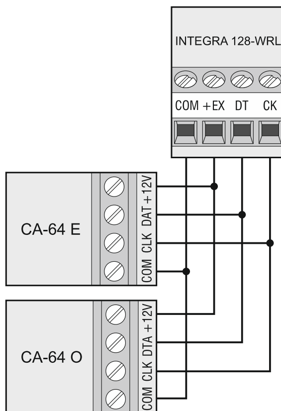
Rys. 6. Sposób podłączania modułów bez zasilacza.
