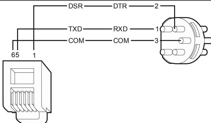
Rys. 16. Sposób podłączenia drukarki za pośrednictwem 5-pinowego wtyku DIN (widok od strony punktów lutowaniczych). Po lewej wtyk RJ podłączany do gniazda na płycie głównej centrali.
